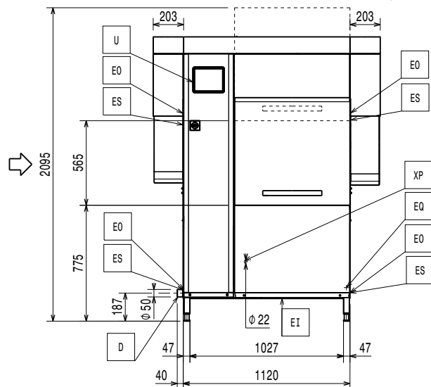
Boční
